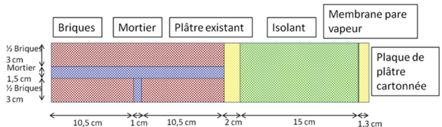
Figure 2 : Schéma de la simulation en 2D de la paroi
