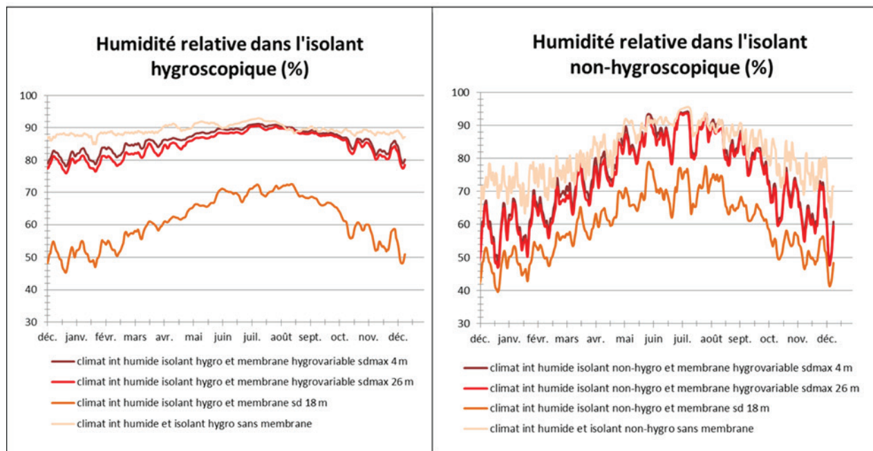
Figure 6 : Climat intérieur humide, humidité relative dans l'isolant
