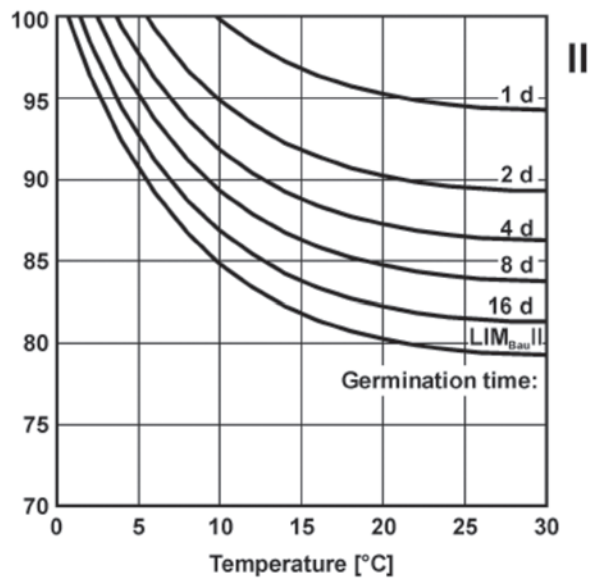
Figure 6 : Zoom sur la germination des spores pour la classe 2 (Sedbauer, 2001), l'axe des ordonnées est en humidité relative et la durée minimum est indiquée sur les courbes en jours (« 16 d » pour 16 jours)
