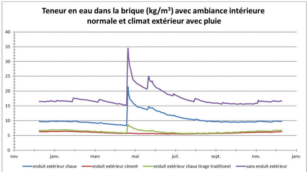
Figure 27 : Teneur en eau dans la brique avec ambiance intérieure normale et climat extérieur avec pluie
