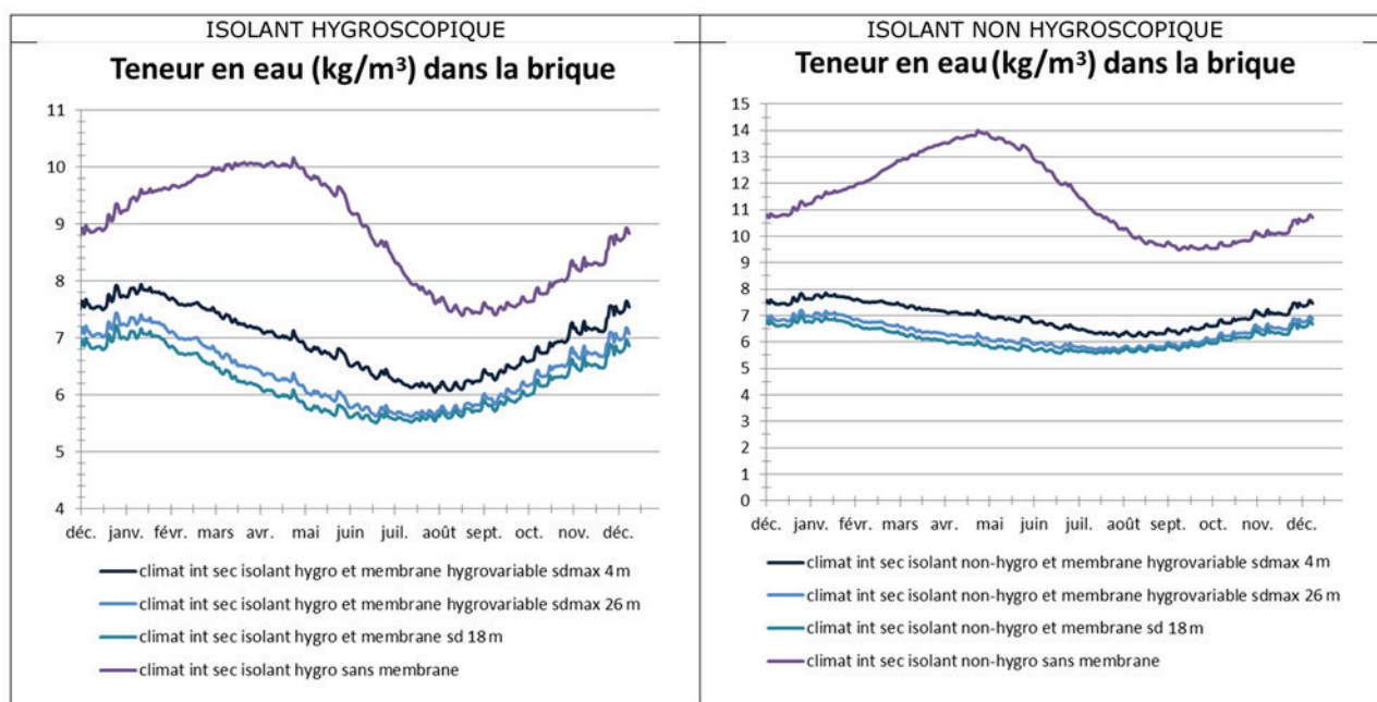
Figure 44 : Climat intérieur normal, teneur en eau dans la brique
