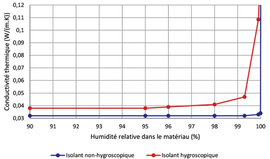
Figure 33 : Conductivité thermique type en fonction de l'humidité relative pour un isolant non-hygroscopique et un isolant hygroscopique (ces courbes ne sont pas uniques et dépendent des produits considérés, elles sont présentées ici à titre d'exemple)
