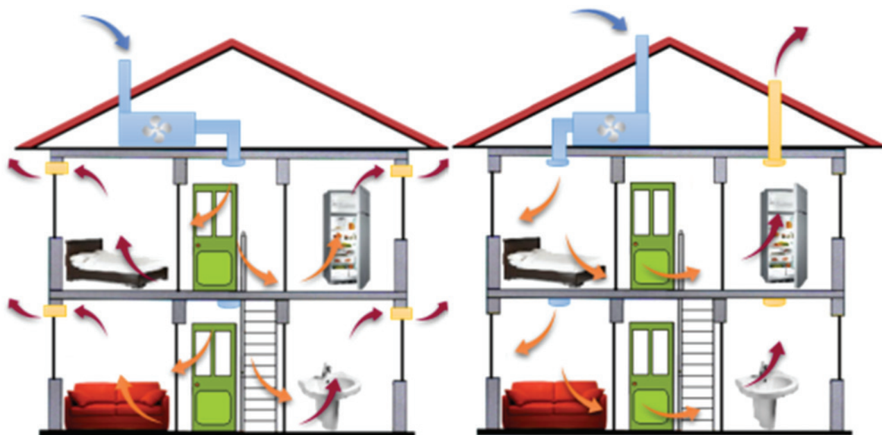
Insufflation centrale Évacuation naturelle via des réglottes
