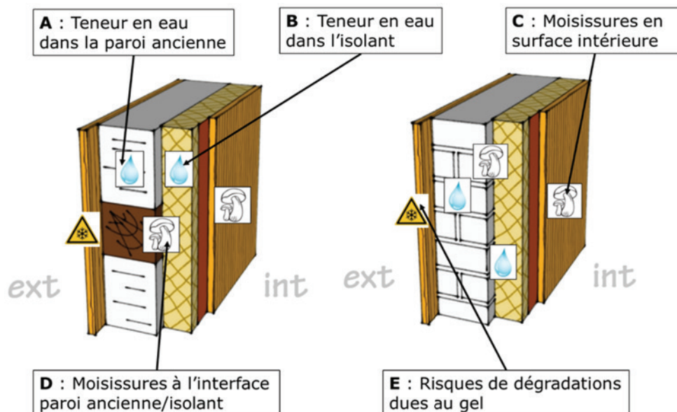
Figure 48 : Indicateurs HUMIBATex
