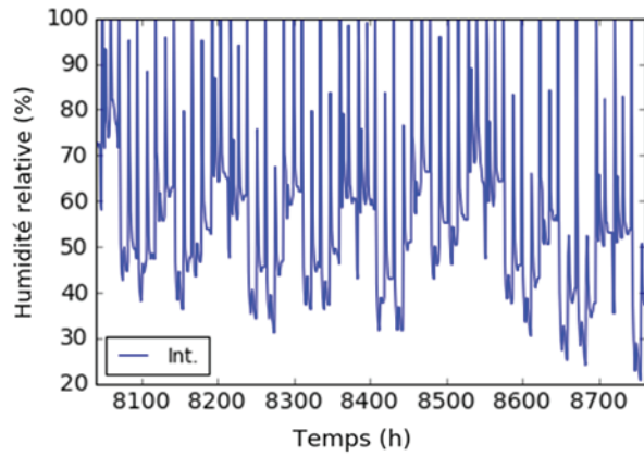
Figure 2 : Évolution de l'humidité relative au niveau de la surface intérieure, paroi en brique isolée par l'intérieur (isolant non hygroscopique) avec présence d'un pare-vapeur ( S_d=18\text{ m} ), climat extérieur : Nancy
