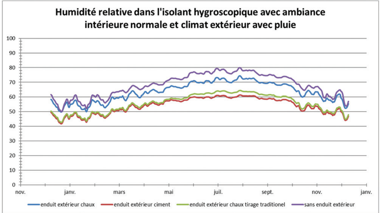
Figure 26 : Humidité relative dans l'isolant hygroscopique avec ambiance intérieure normale et climat extérieur avec pluie
