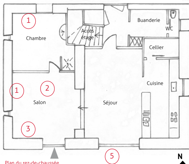
Plan du rez-de-chaussée après travaux
